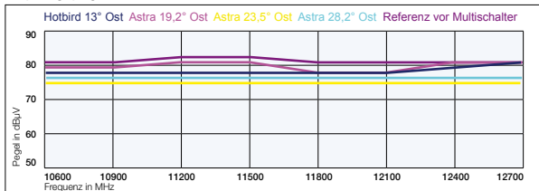
Empfangspegel
